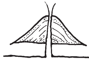
B. GRANITIC
